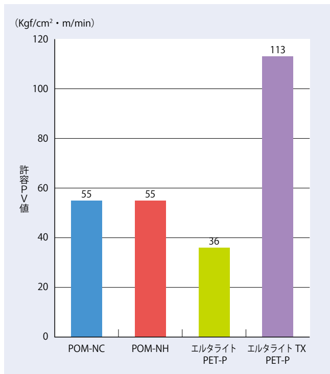
許容PV値比較 (速度:30m/min)
