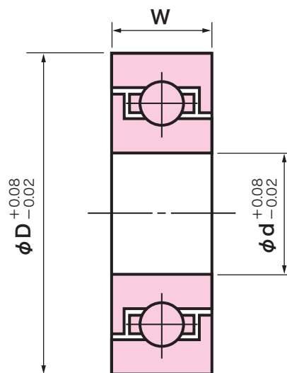
タイプ-P
