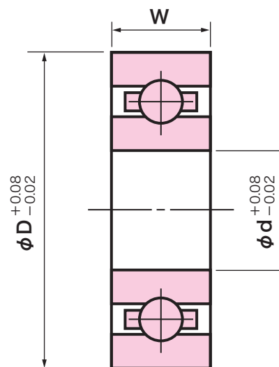
タイプ-N
